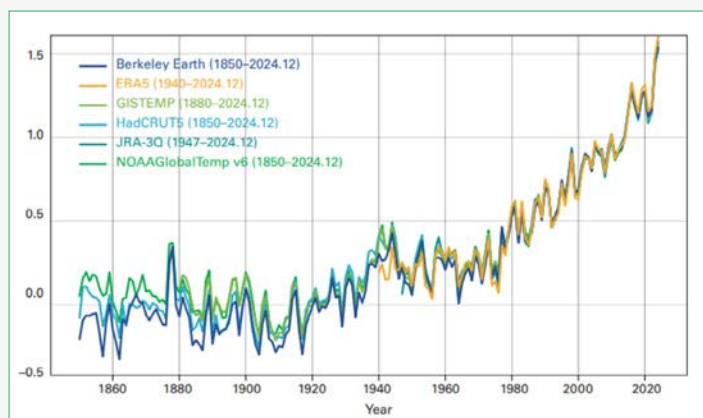
全球年平均气温异常值（相对于工业化前基准线，时间范围：1850—2024 年）
